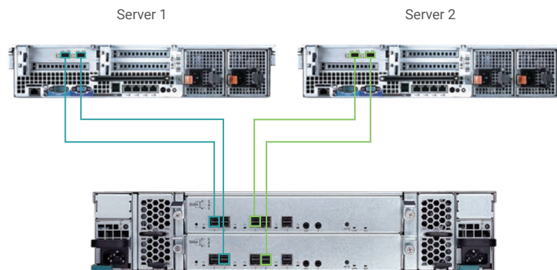
Topologia MPIO ad alta disponibilità per server cluster
